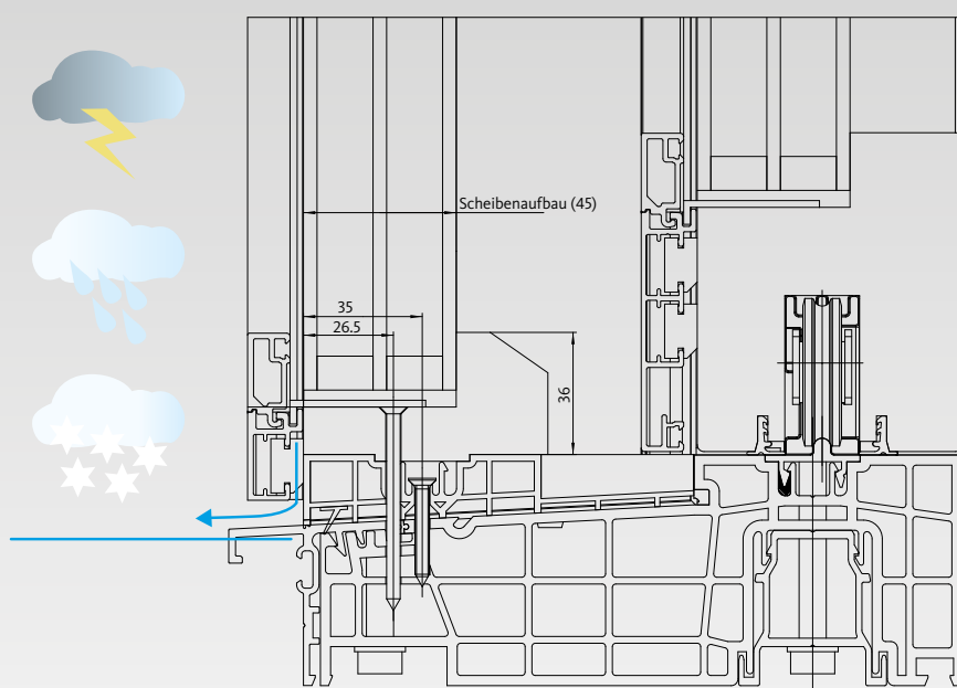
Querschnitt im Festfeldbereich
